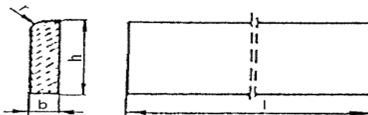
Rysunek 1. Kształt betonowego obrzeża chodnikowego.
