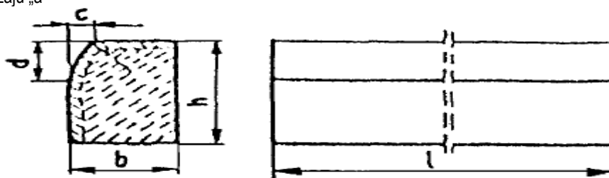
Rys. 1. Wymiarowanie krawężników
