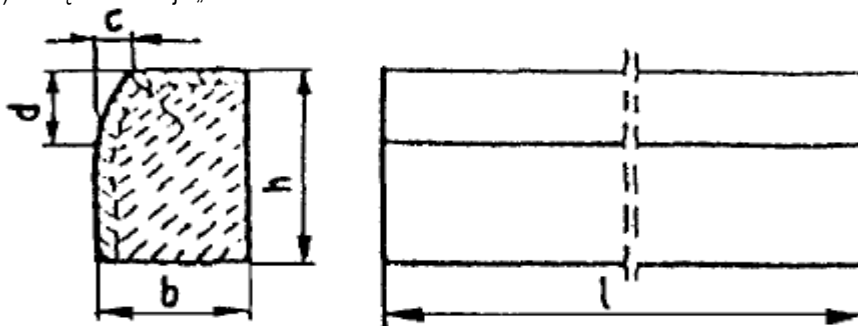
Rys. 1. Wymiarowanie krawężników
